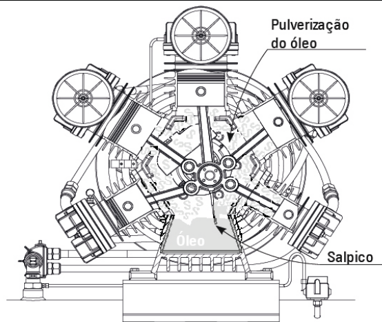
Figura 9 Lubrificação Interna
